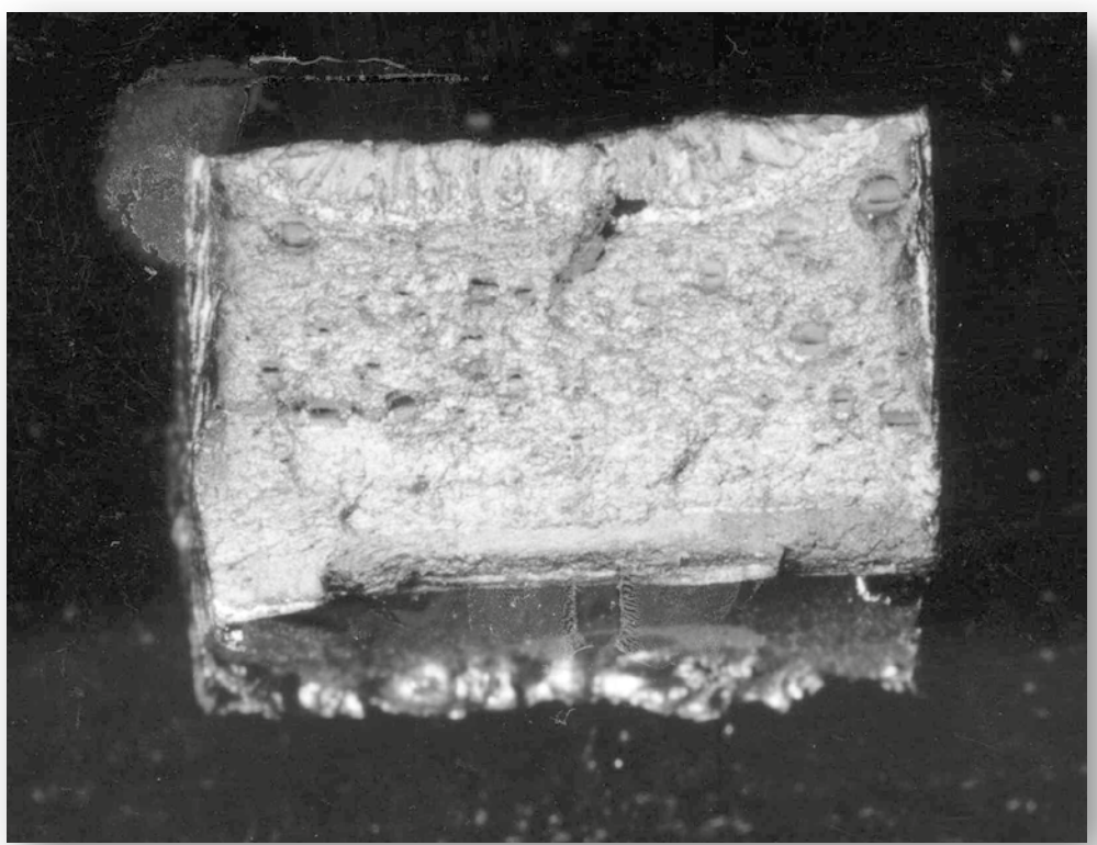
Erstarrungsrisse
