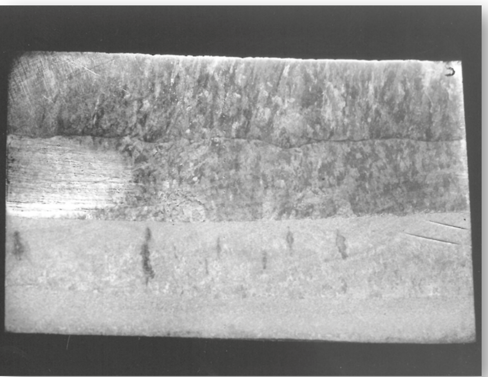
Wiederaufschmelzungsrisse
