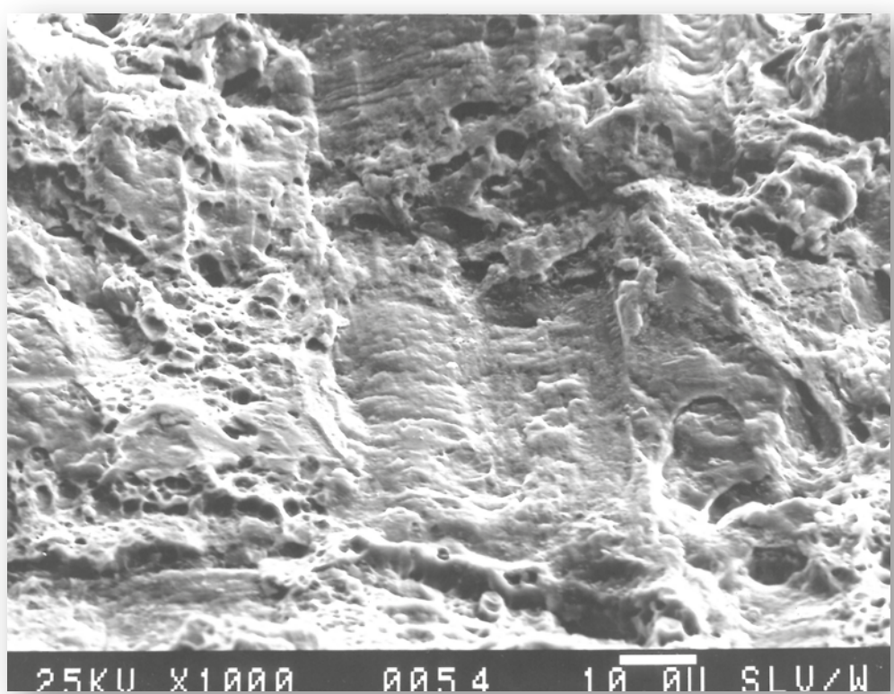
Schwingungsbruch
