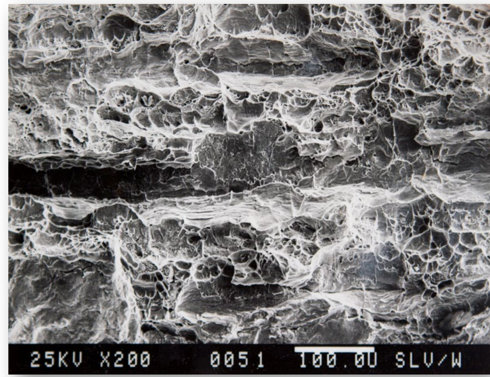
Terrassenbruch
