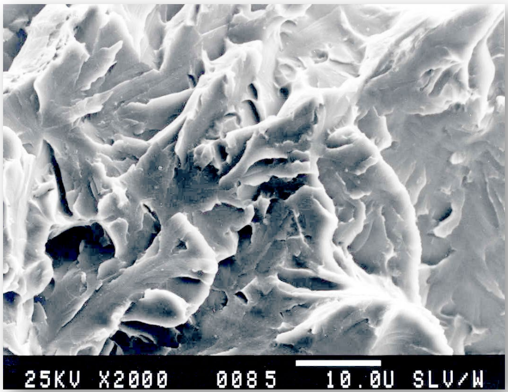
transkristalline H 2 -Versprödung
