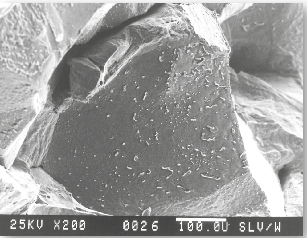
Wiederaufschmelzungsrisse
