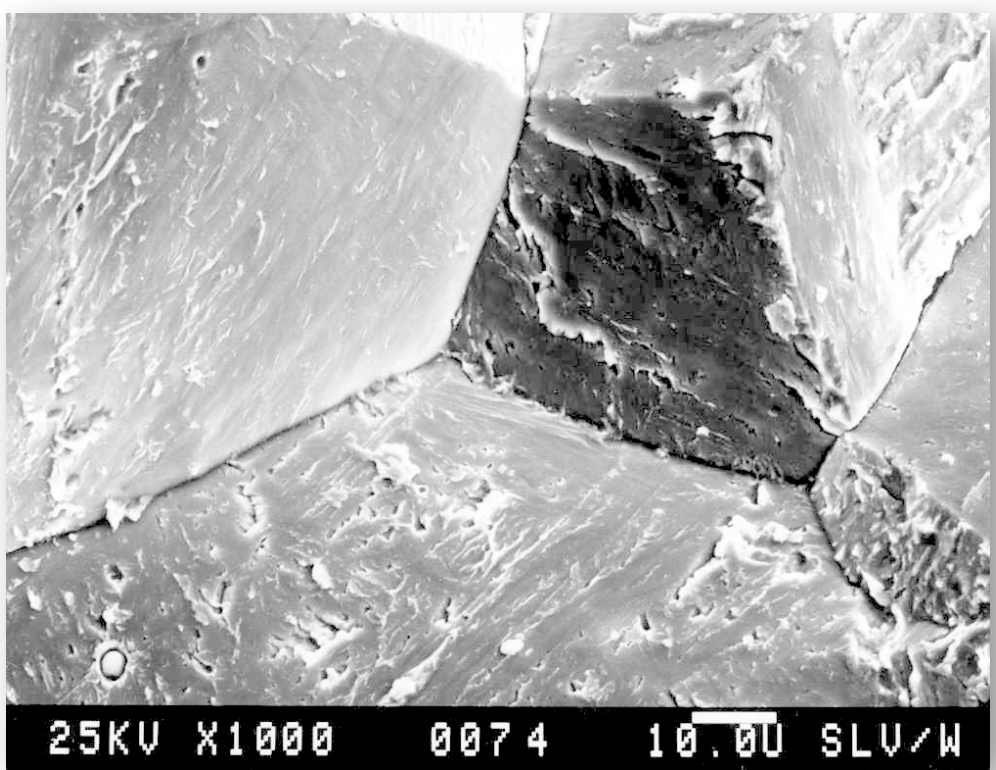
interkristalline H 2 -Versprödung
