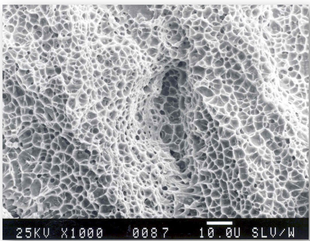
duktiler Gewaltbruch
