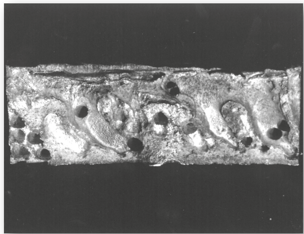
mechanische Pore
