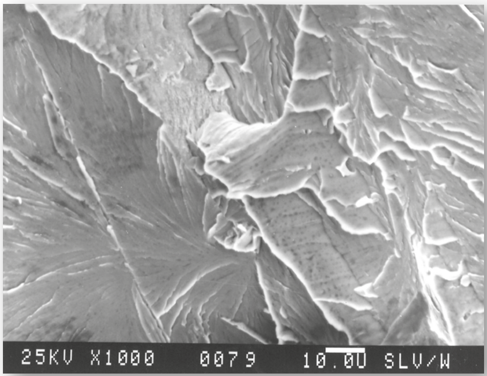
transkristalliner Aufhärtungsrisse
