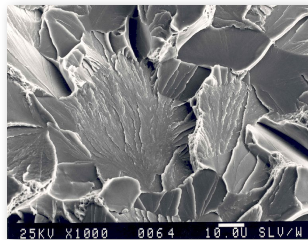
transkristalliner Gewaltbruch
