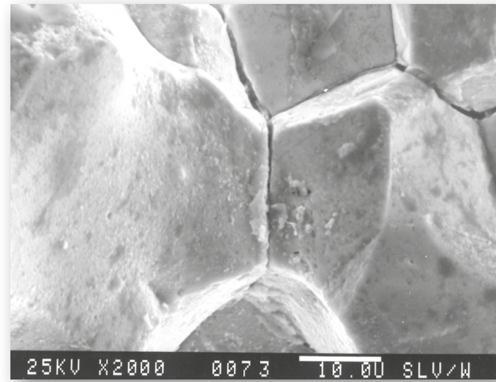
Unterplattierungsrisse
