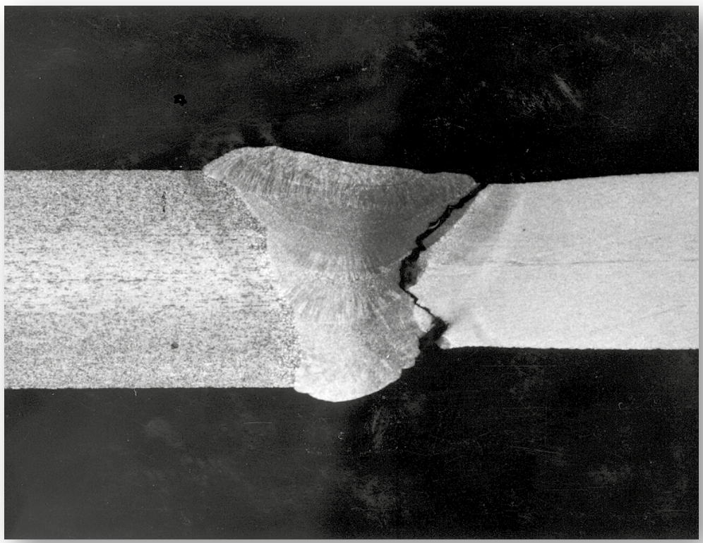
H 2 -induzierte Risse
