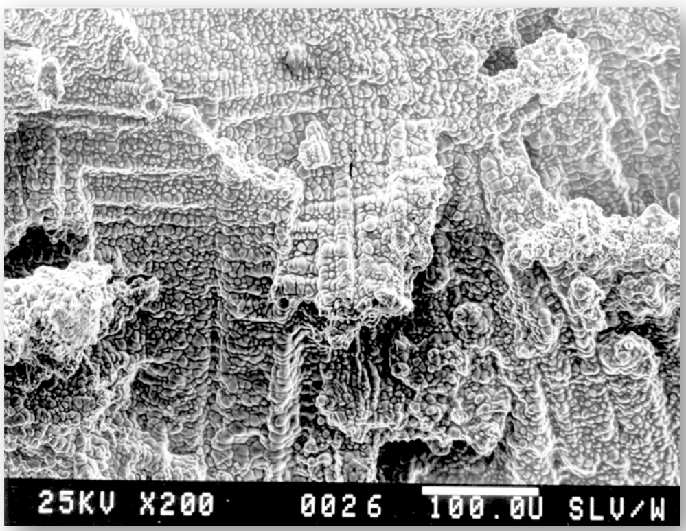
Erstarrungsrisse
